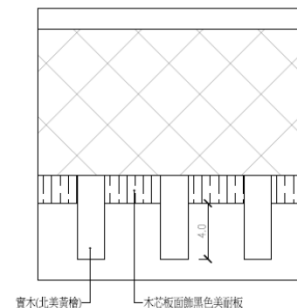
② 海運辦公室大廳木格柵造型大樣圖 S:1/2CM
