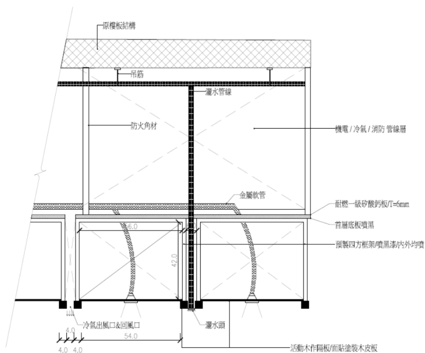
① 海運辦公室大廳及大會議室天花板造型大樣圖 S:1/10CM
