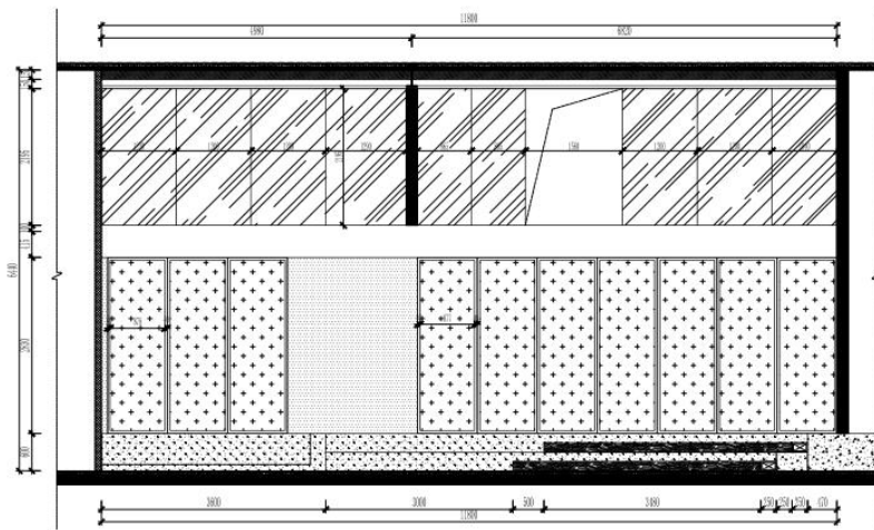
05 ORIGINAL STRUCTURE PLAN 一层中庭立面 SCALE: 1/60
