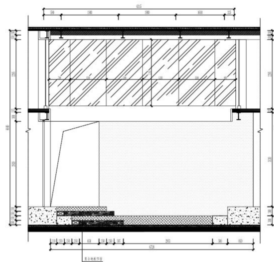
05 ORIGINAL STRUCTURE PLAN 一层中庭立面 SCALE: 1/60
