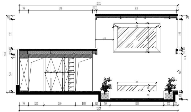
05 ORIGINAL STRUCTURE PLAN 一层中庭B立面 SCALE: 1/60
