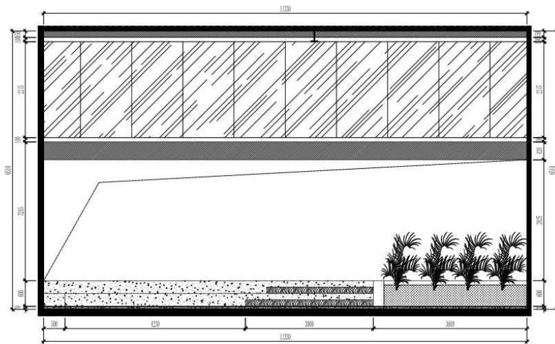
05 ORIGINAL STRUCTURE PLAN 一层中庭A立面 SCALE: 1/60
