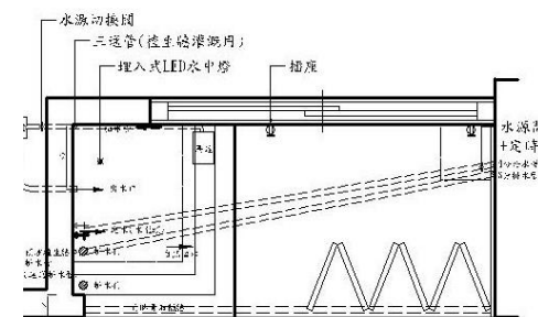
造景配管標示圖
