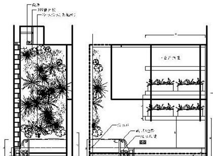
造景左側立視圖
