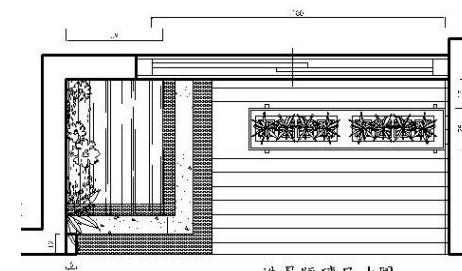
造景隔磚尺寸圖
