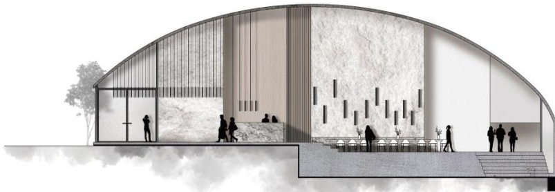
AA' 剖立面圖
